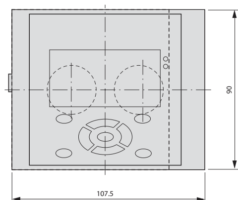
MFD-80... + MFD-CP... + MFD-R.../MFD-T... MFD-80... + MFD-AC-CP... + MFD-AC-R16
